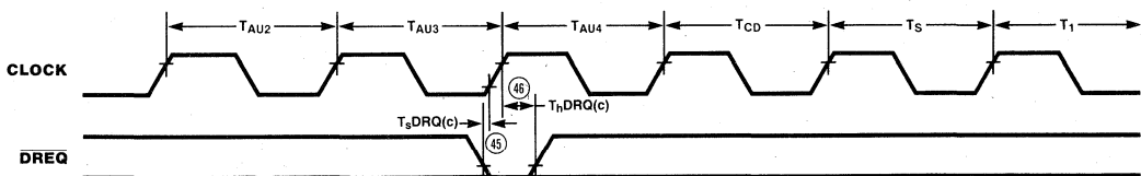
(D) Sampling \overline{\text{DREQ}} at End of Base-to-Current Reloading
